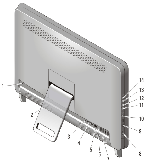
Figura 2. Vista traseira
